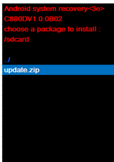
图 3-5 SD 卡目录
